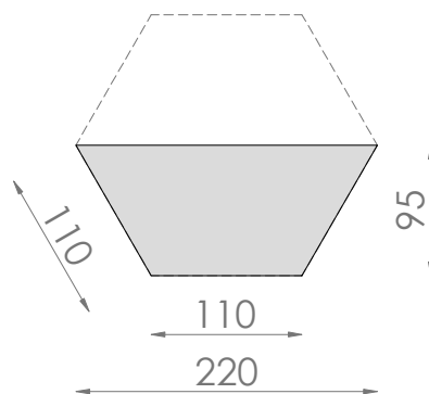
8.03.1.4. Płyta H06S2 / 0,016m 2
