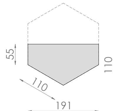
8.03.1.5. Płyta H06S3 / 0,016m 2
