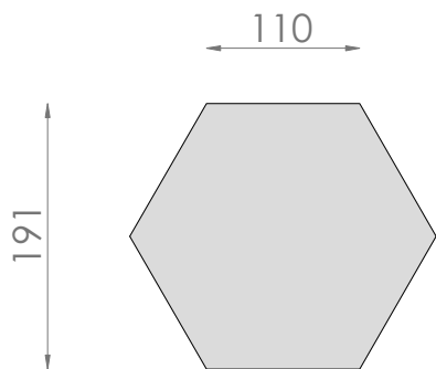
8.03.1.1. Płyta H06 / 0,03m 2
