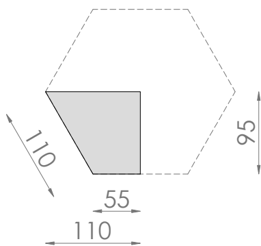
8.03.1.3. Płyta H06S1 / 0,008m 2
